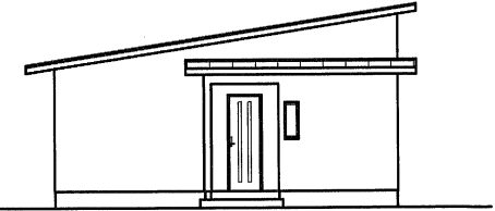
東側 立面図
