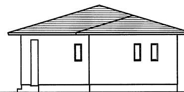
東側 立面図
