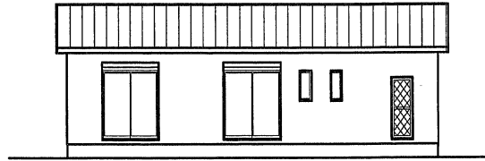
南側 立面図
