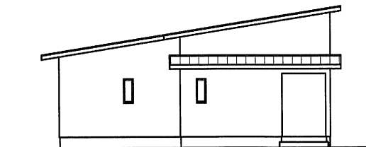
西側 立面図
