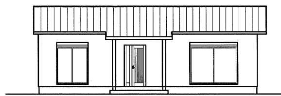
南側 立面図
