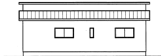
北側 立面図
