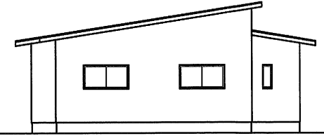
東側 立面図
