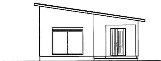
南側 立面図
