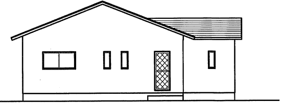
東側 立面図
