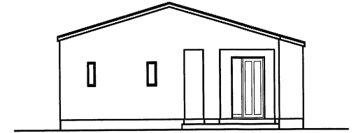
東側 立面図
