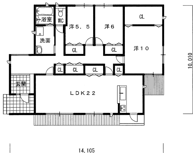
平面図
