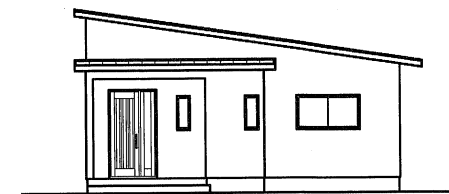
東側 立面図
