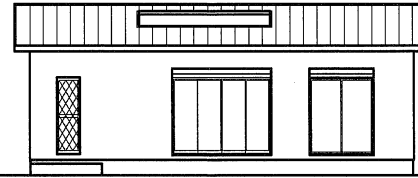
南側 立面図
