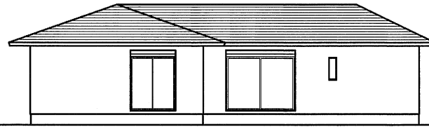
南側 立面図
