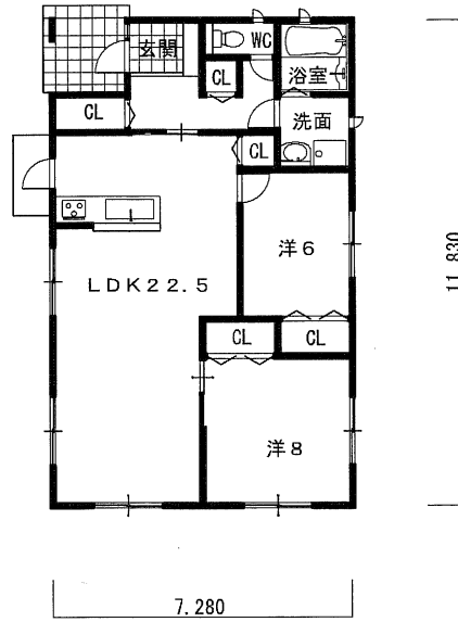
平面図
