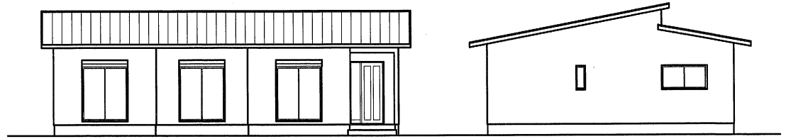
南側 立面図
