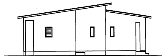
東側 立面図
