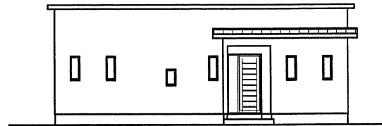
北側 立面図
