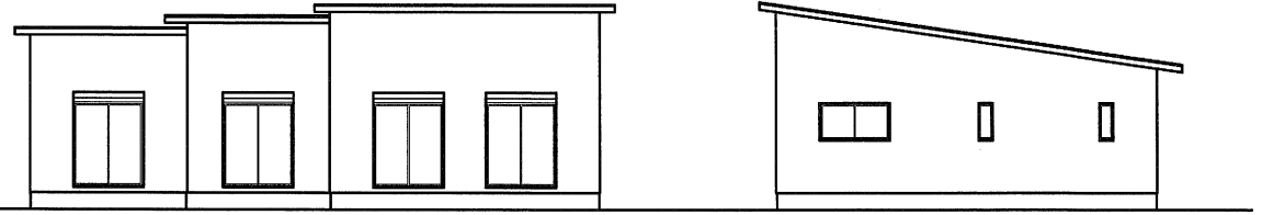
南側 立面図
