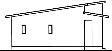
東側 立面図
