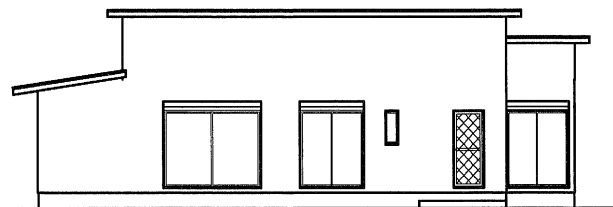
南側 立面図
