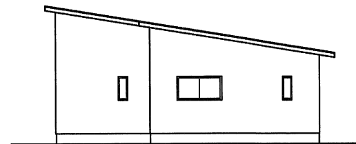
東側 立面図
