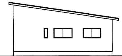
西側 立面図
