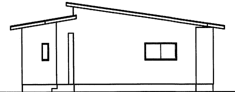
西側 立面図
