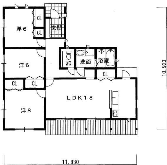
平面図
