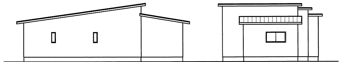
北側 立面図
