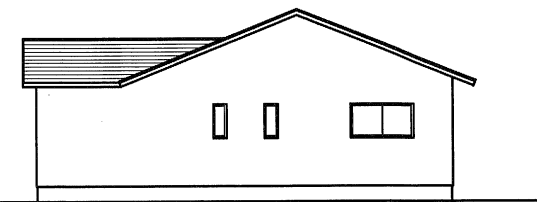
西側 立面図
