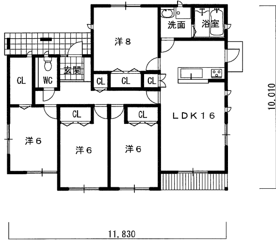
平面図
