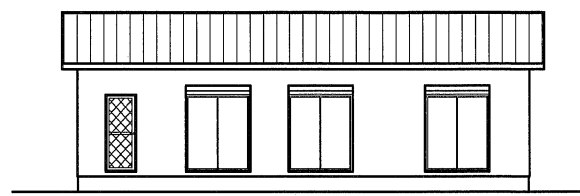
南側 立面図
