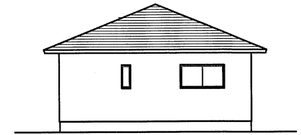
東側 立面図
