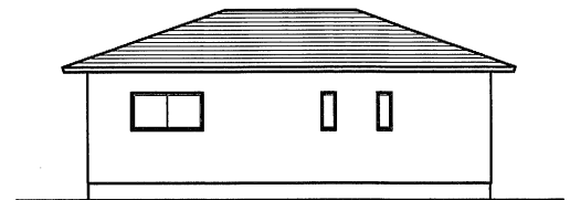
西側 立面図
