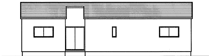
北側 立面図
