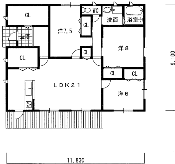
平面図
