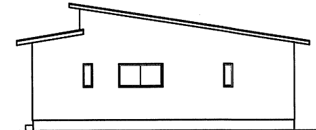
西側 立面図
