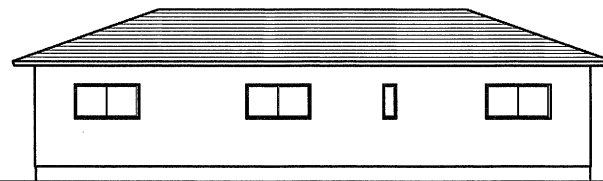
北側 立面図
