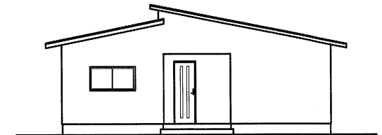
西側 立面図
