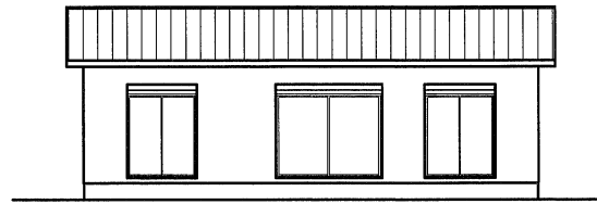
南側 立面図
